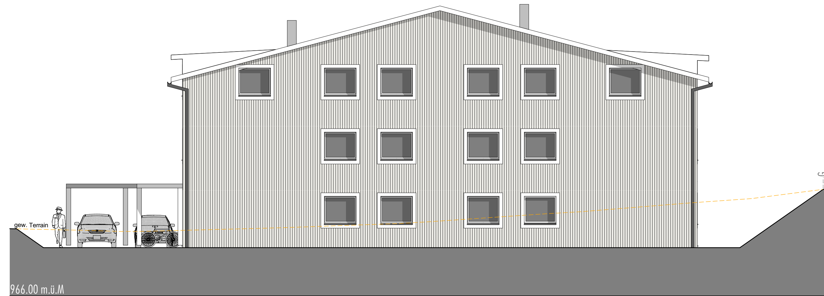
966.00 m.ü.M Ansicht Nord-West
